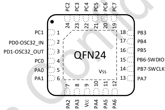
图 3-5 QFN24 Pinout1 PY32F005E1xU7
