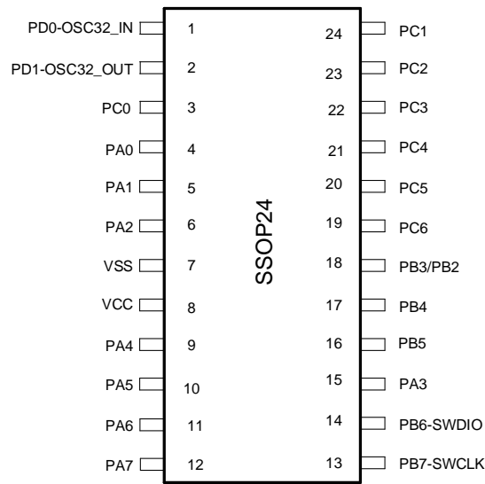
图 3-2 SSOP24 Pinout1 PY32F005E1xM7
