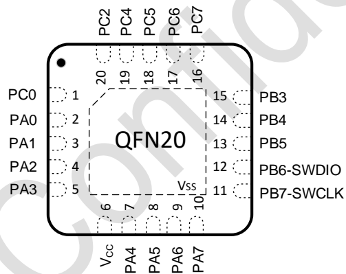
图 3-6 QFN20 Pinout1 PY32F005F1xU7
