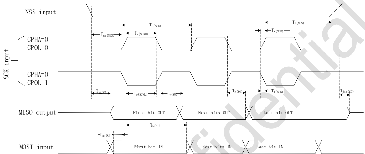
图 5-4 SPI 时序图 – 从机模式, CPHA=0
