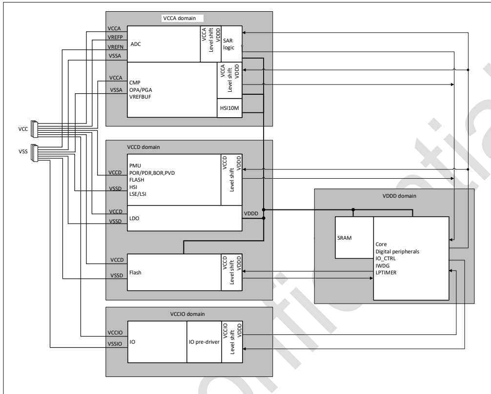
图 2-2 电源框图
