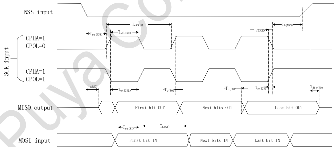
图 5-5 SPI 时序图 – 从机模式, CPHA=1
